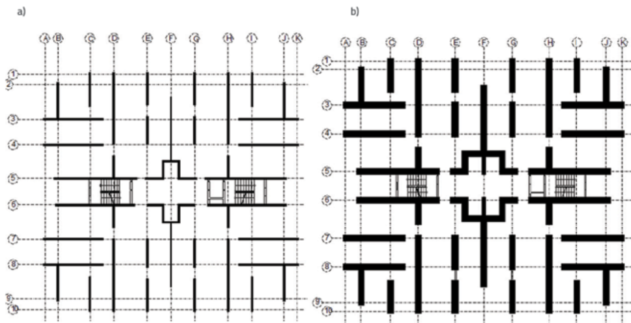
Slika 1. Tlocrtni prikaz građevine: tlocrt s dva dizala, b) tlocrt s četiri dizala
