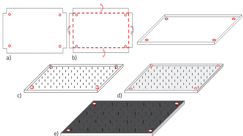
Slika 6. Skica slijeda proizvodnje za montažne spregnute ploče: a) i b) Savijanje posebno oblikovane čelične ploče debljine 2 \text{ mm} ; c) ploča sa zavarenim posmičnim moždanicima i rupicama na uglovima, izbušenim za pričvršćivanje, okružena cilindričnim cijevima; d) ugradnja betona; e) postavljanje gornje ploče sa zavarenim posmičnim moždanicima
