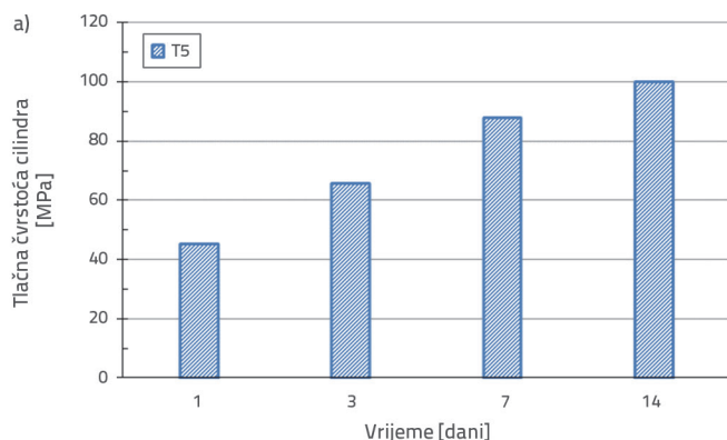
Slika 4. a) Vrijednosti tlačne čvrstoće skupa valjkastih uzoraka dobivenih iz mješavine T5; b) Ispitivanje mješavine T5 pomoću lijevka koje pokazuje slijevanje od 4 cm
