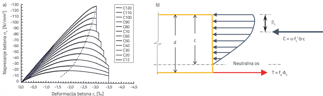
Slika 8. a) Krivulje napreznje – deformacija za različite klase čvrstoće betona [23]; b) skica raspodjele tlačnih napreznja u betonu i vlačnih napreznja u čeliku u poprečnom presjeku
