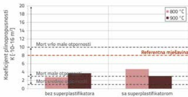
Slika 7. Koeficijent plinopropusnosti ispitivanih mortova s ugrađenim pepelom
