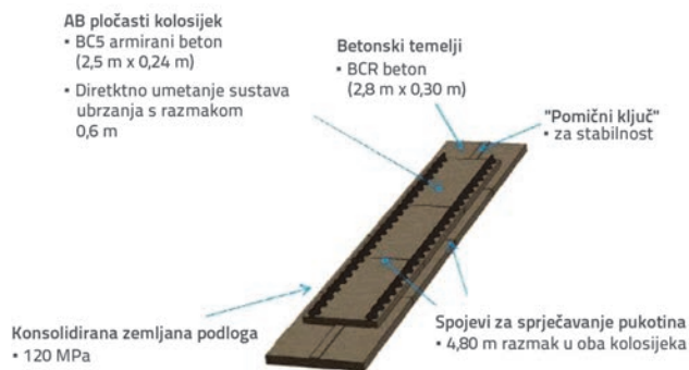
Slika 9. Shema NBT - novog kolosijeka bez zastorne prizme
