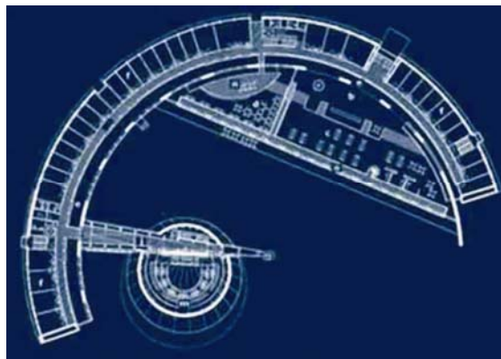
Tlocrt nove zgrade samskoga parlamenta
